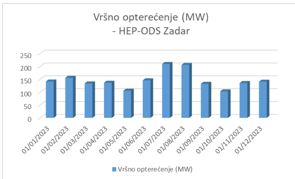
Slika 3 Vršno opterećenje HEP-ODS Zadar
