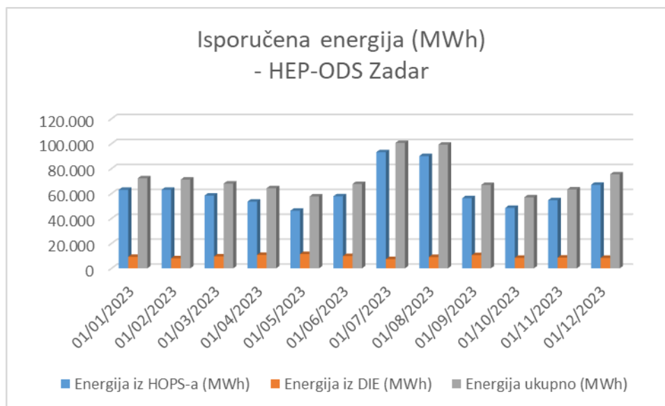
Slika 2 Isporučena energija HEP-ODS Zadar
