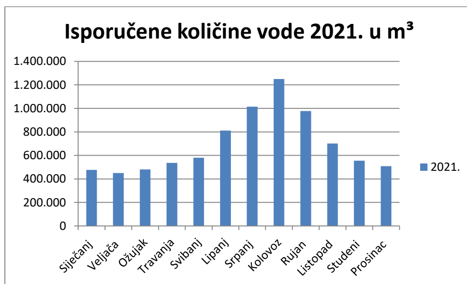
Slika 6 Sezonska varijabilnost u potrošnji vode na uslužnom području Vodovoda d.o.o. Zadar 2021. Godine
